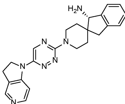
( S )-1'-(6-(2,3-dihydro-1 H -pyrrolo[3,2- c ]pyridin-1-yl)-1,2,4-triazin-3-yl)-1,3-dihydrospiro[indene-2,4'-piperidin]-1-amine
