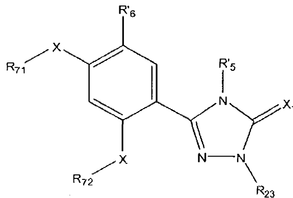
(XVI)
