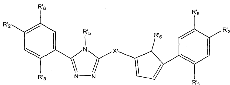
(XIV)
