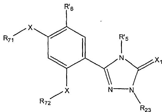
(XVI)
