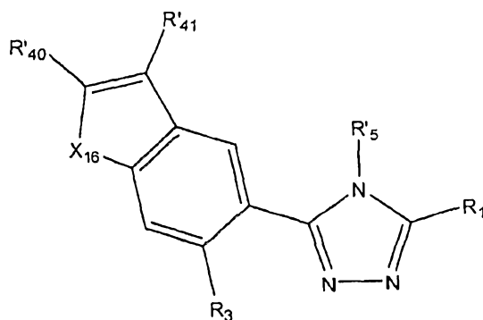
(XXII)
