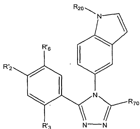
(XV)
