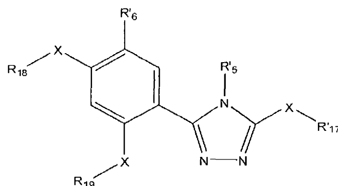
(XI)
