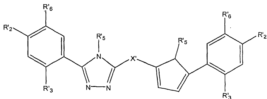
(XIV)
