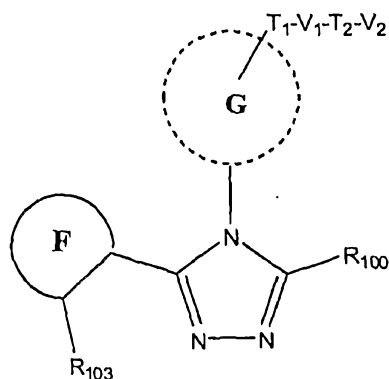
(XXVIII)
