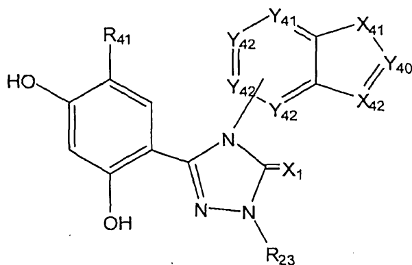
(XVIII)
