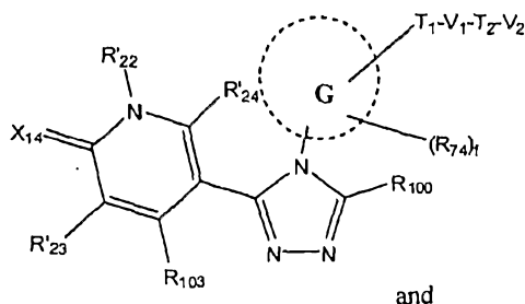
(XXIX)
