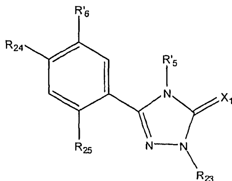
(XVII)
