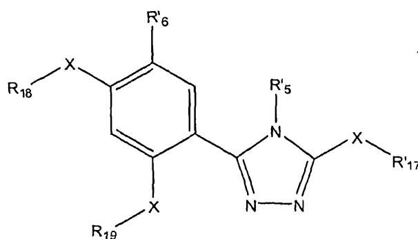
(XI)
