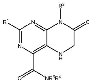
(IIId)
