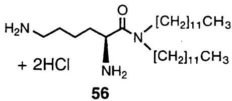
N 1 ,N 1 -dioctadecyl-1,2,6-triaminohexane tri HCl salt
