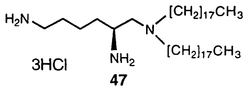
N 1 ,N 1 -dioctadecyl-1,2,6-triaminohexane tri HCl salt
