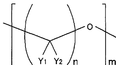
[Chem. Formula 3]
