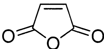
Maleic anhydride
