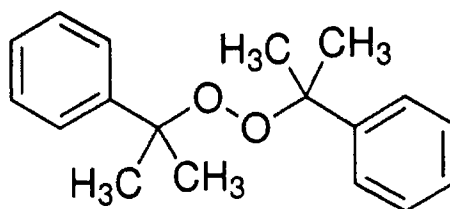
Dicumyl peroxide
