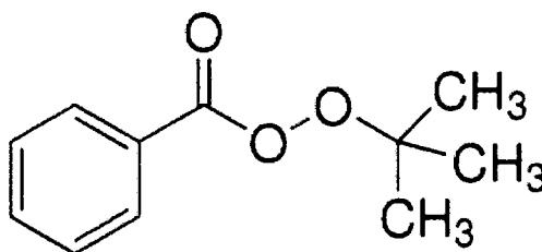
tert-Butyl peroxybenzoate
