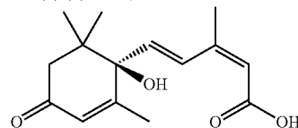
(R)-(-)-2-cis-,4-trans-abscisic acid
