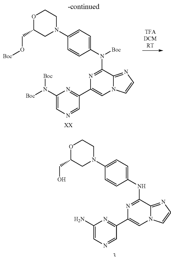
(R)-(4-(4-((6-Bromoimidazo[1,2-a]pyrazin-8-yl)amino)phenyl)morpholin-2-yl)methanol XVII
