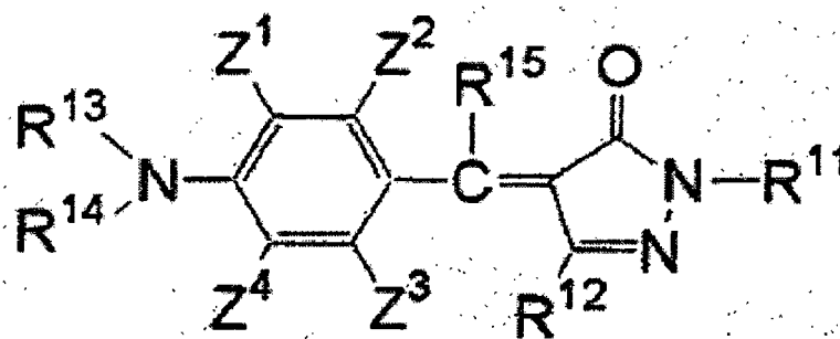
Formule (II)
