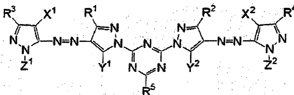
Formule (I)
