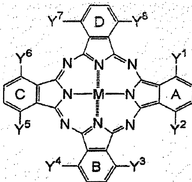
Formule (VII)
