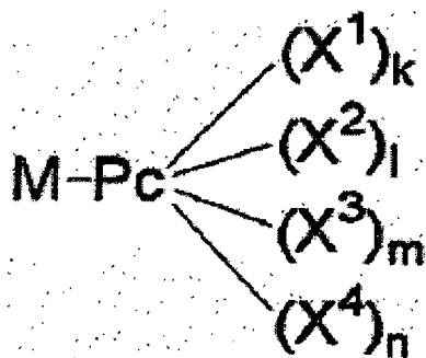
Formule (VI)
