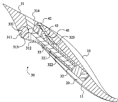
SECTION D-D
