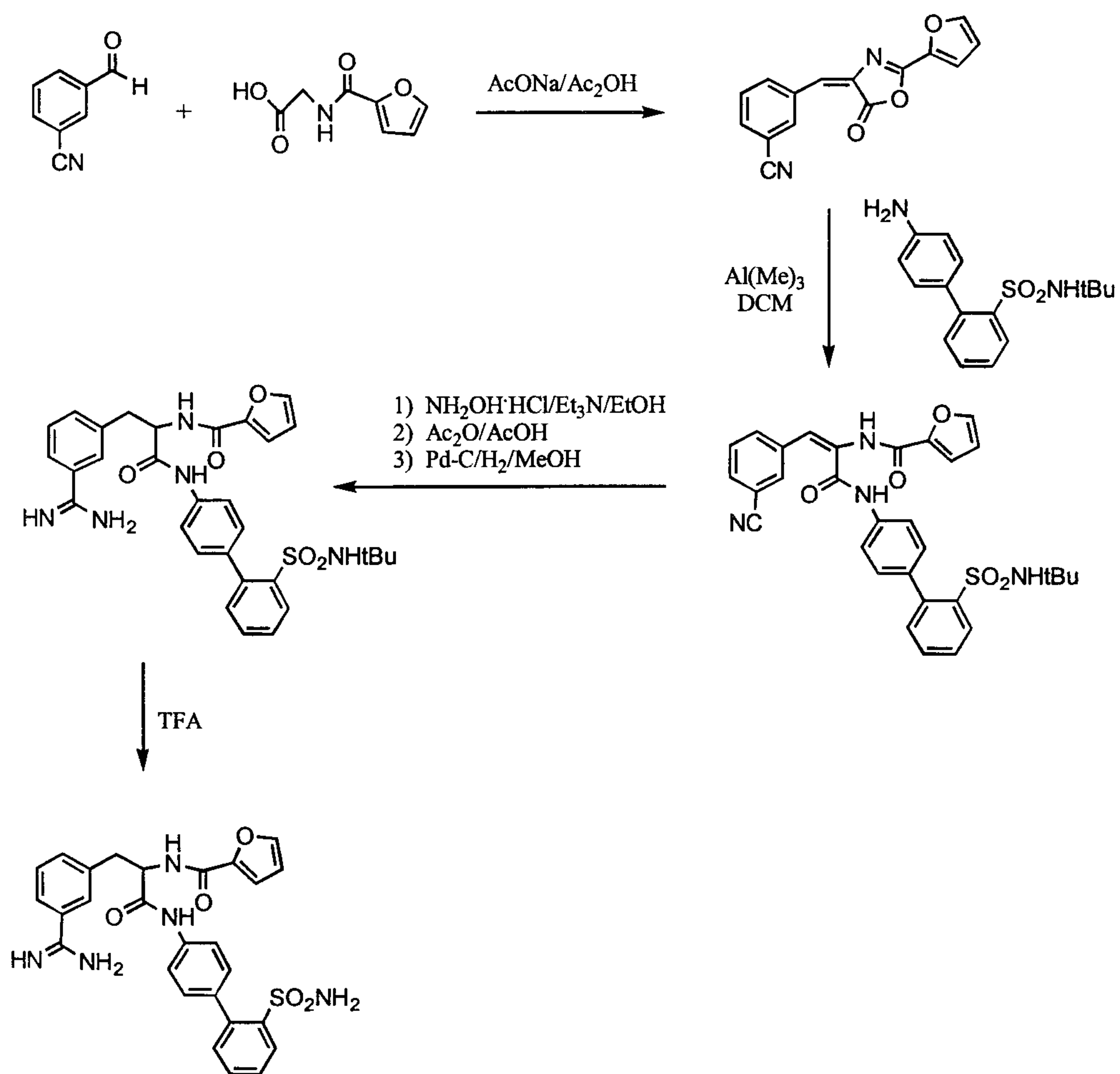
Scheme3
