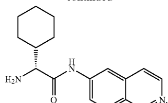
(R)-2-amino-2-cyclohexyl-N-(isoquinolin-6-yl)acetamide
