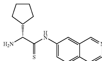
(R)-2-amino-2-cyclopentyl-N-(isoquinolin-7-yl)acetamide
