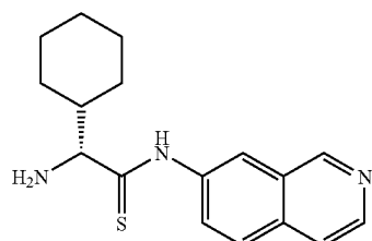
(R)-2-amino-2-cyclohexyl-N-(isoquinolin-7-yl)acetamide
