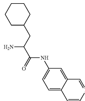
2-amino-3-cyclohexyl-N-(isoquinolin-7-yl)propanamide
