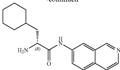
(R)-2-amino-3-cyclohexyl-N-(isoquinolin-7-yl)propanamide
