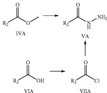
Scheme 2A
