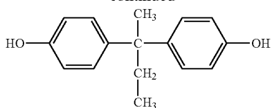
BisP-B
