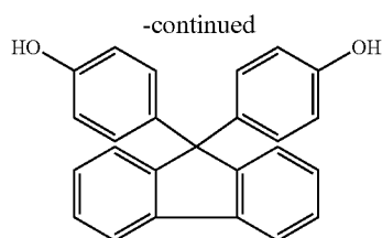
BisP-FL
