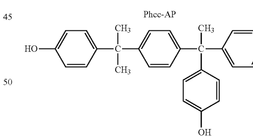
BisP-PA
