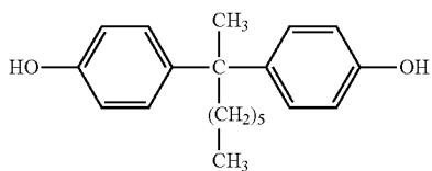
BisP-OT
