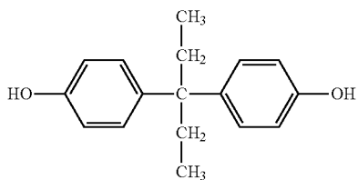
BisP-DEK
