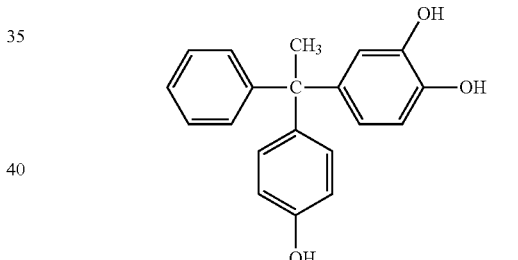
BisP-DP
