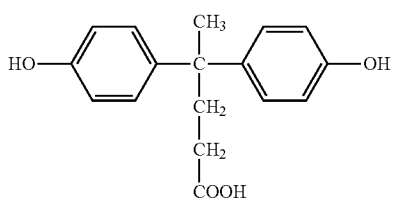
BisP-LV
