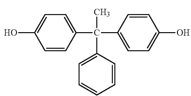
BisP-AP
