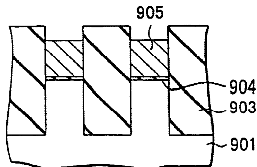
FIG. 14E
