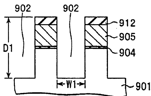
FIG. 14B
