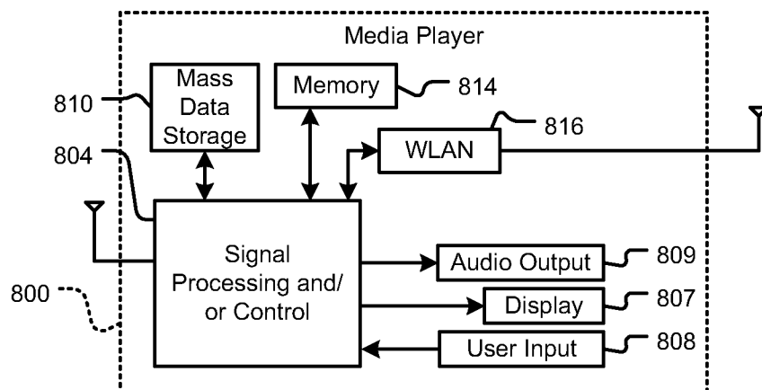
FIG. 7F
