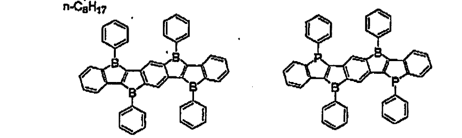
[Chem 15]
