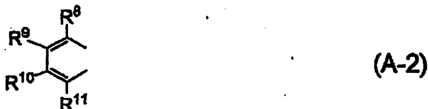
[Chem 3]
