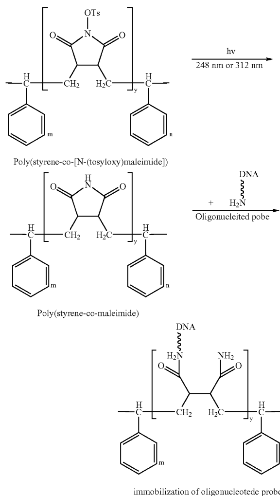
Scheme I:
