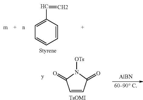
Scheme II:
