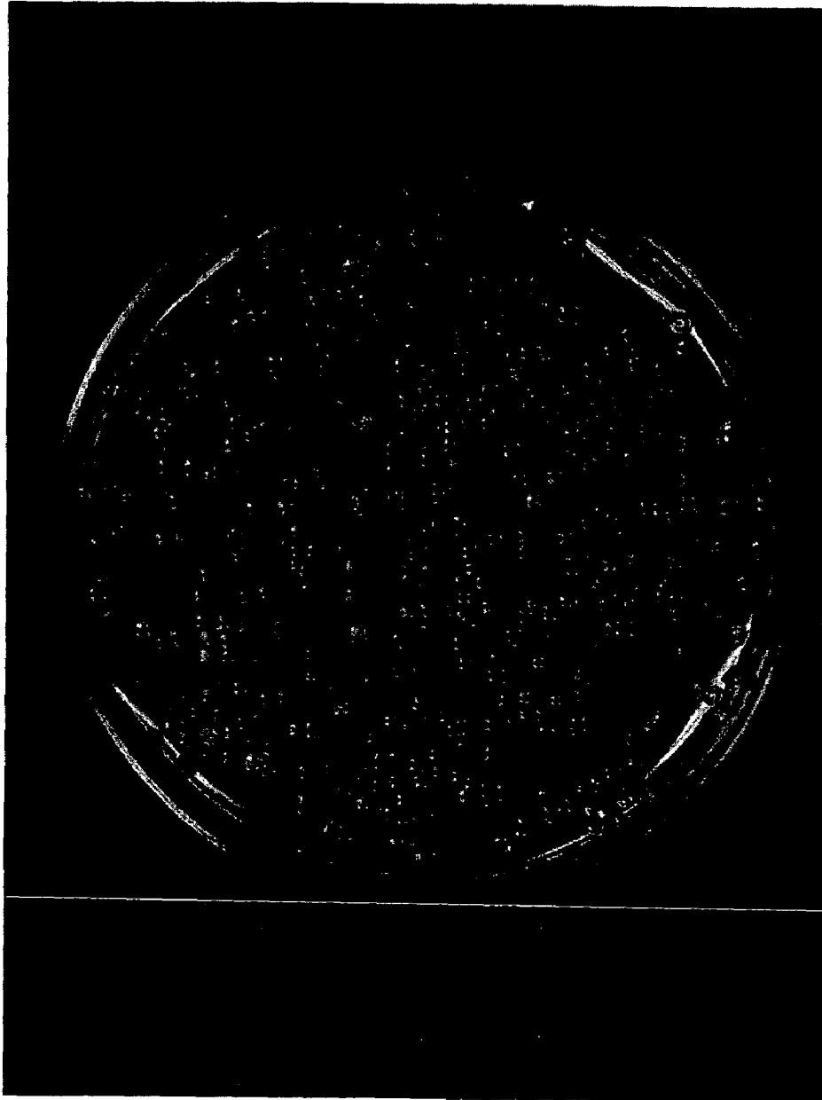
Fig. 3. Ribocloning a Ds-Red gene.
