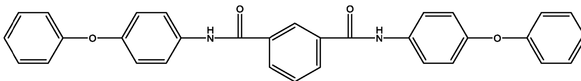
EAm-1,3-AmE
