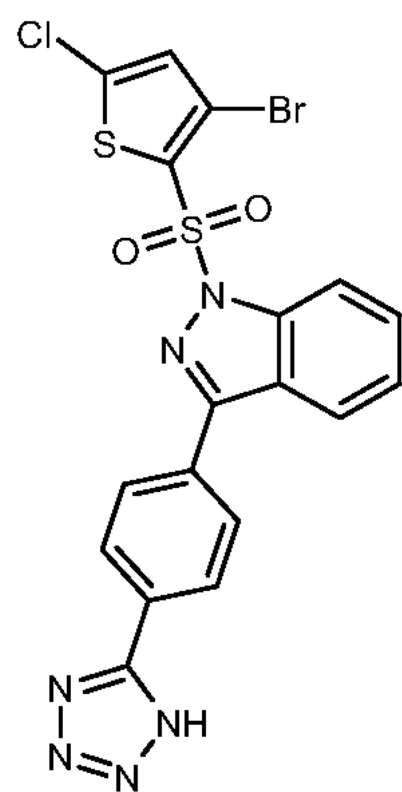
5 21C: 3-(4-(1H-tetrazol-5-yl)phenyl)-1-(3-bromo-5-chlorothiophen-2-ylsulfonyl)-1H-indazole
