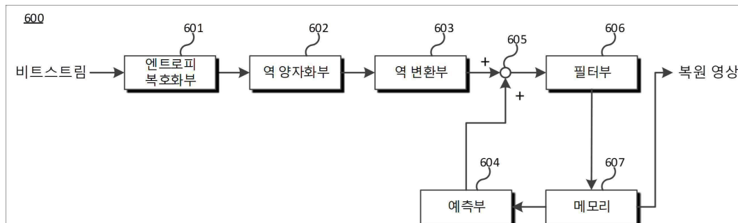
도면7
