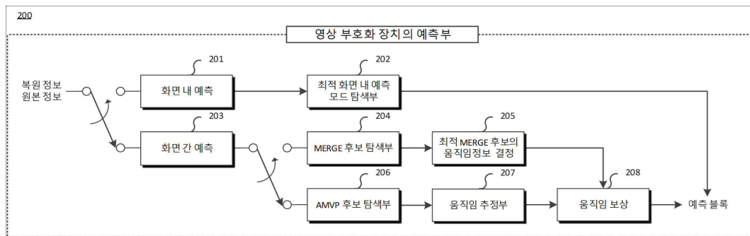
도면2
