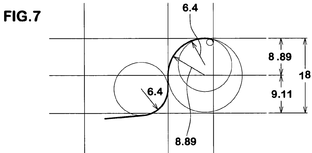
TRA 13-18 RIM DIA. CONTOUR
