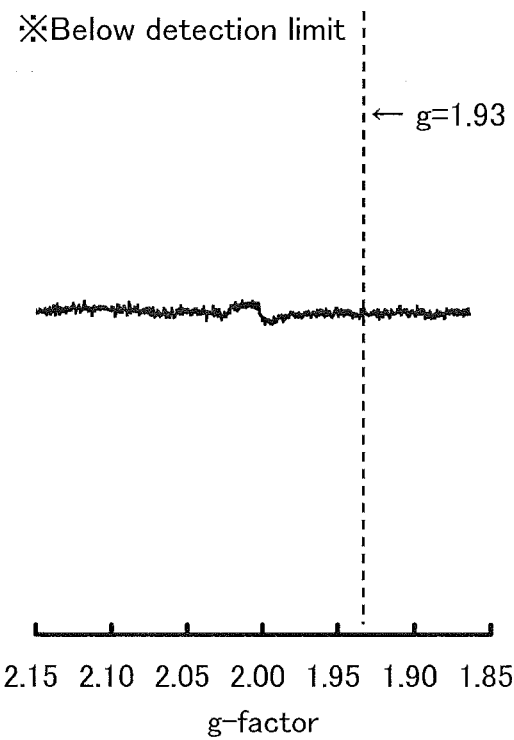
FIG. 28
