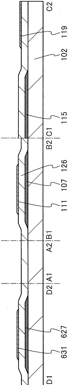
FIG. 4A
