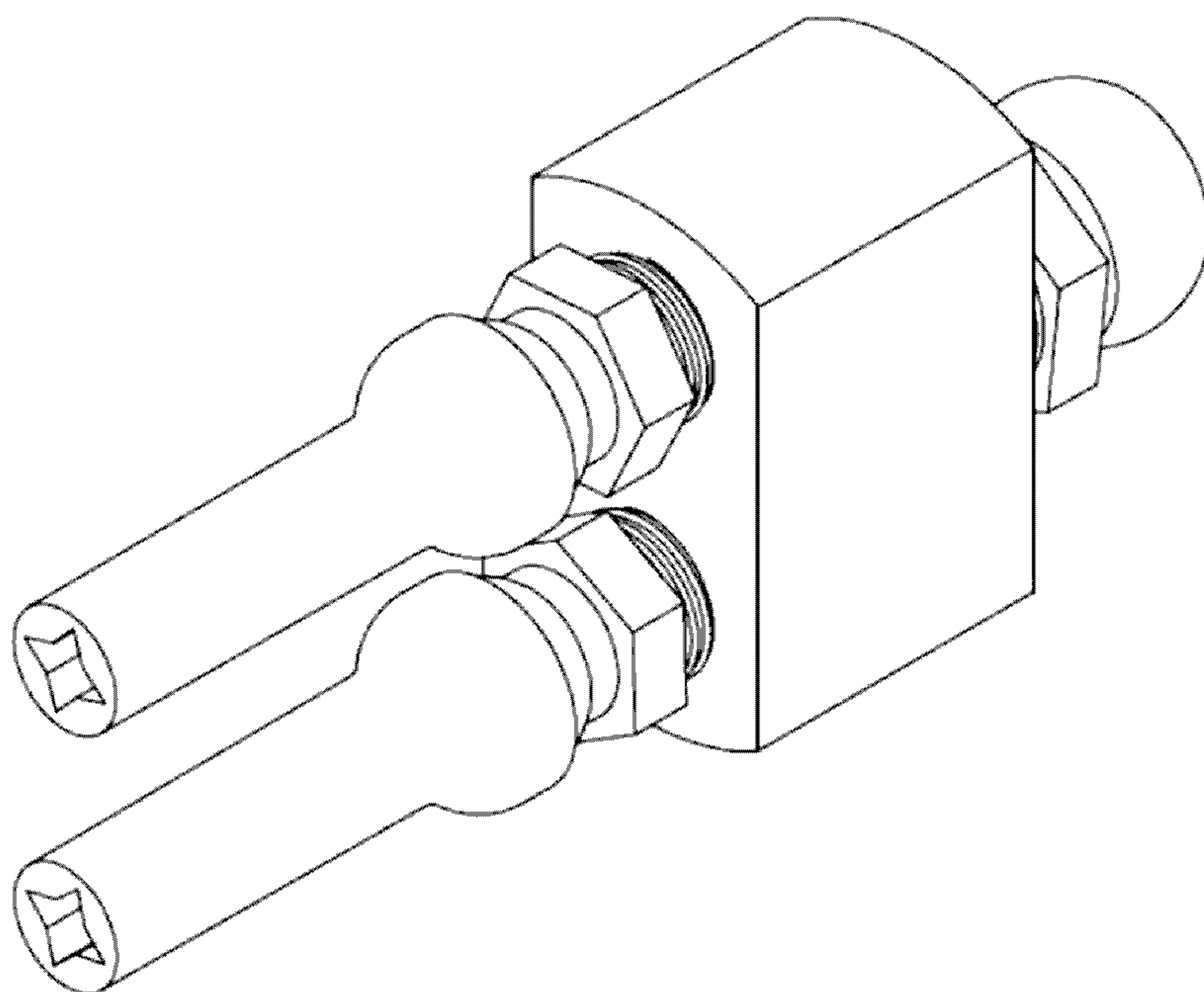
【立體圖 1】
