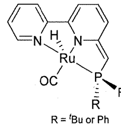
RuPNN-Bipy
