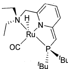
RuPNN-Et 2
