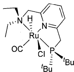
RuPNN-Et 2
