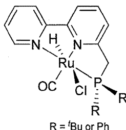
RuPNN-Bipy
