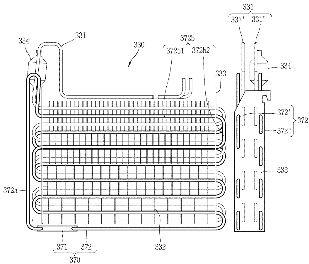
FIG. 11 (b)
