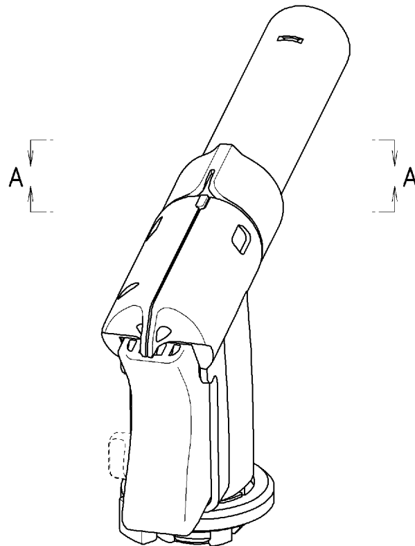
【立體圖3】
