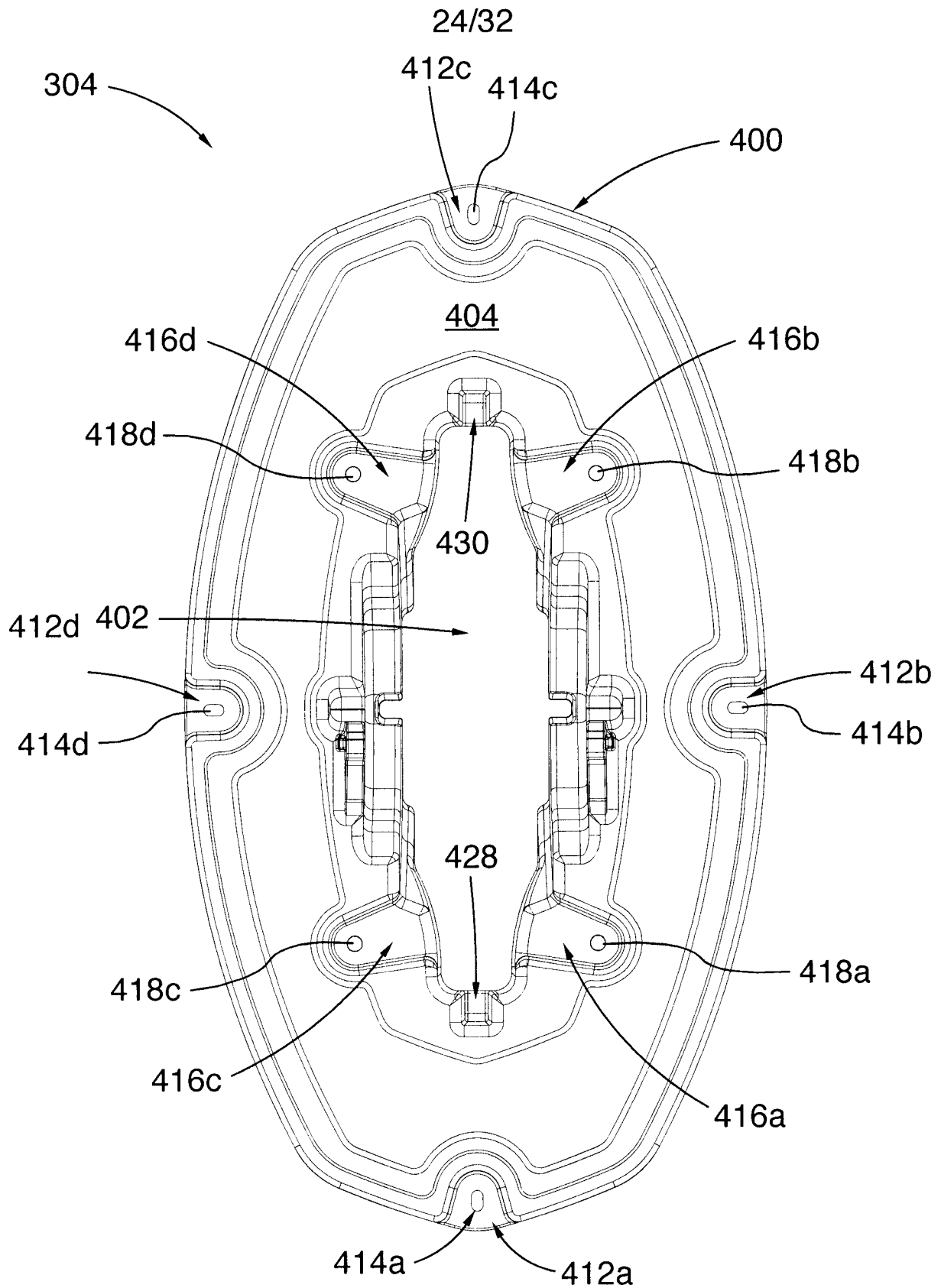
FIG.23
