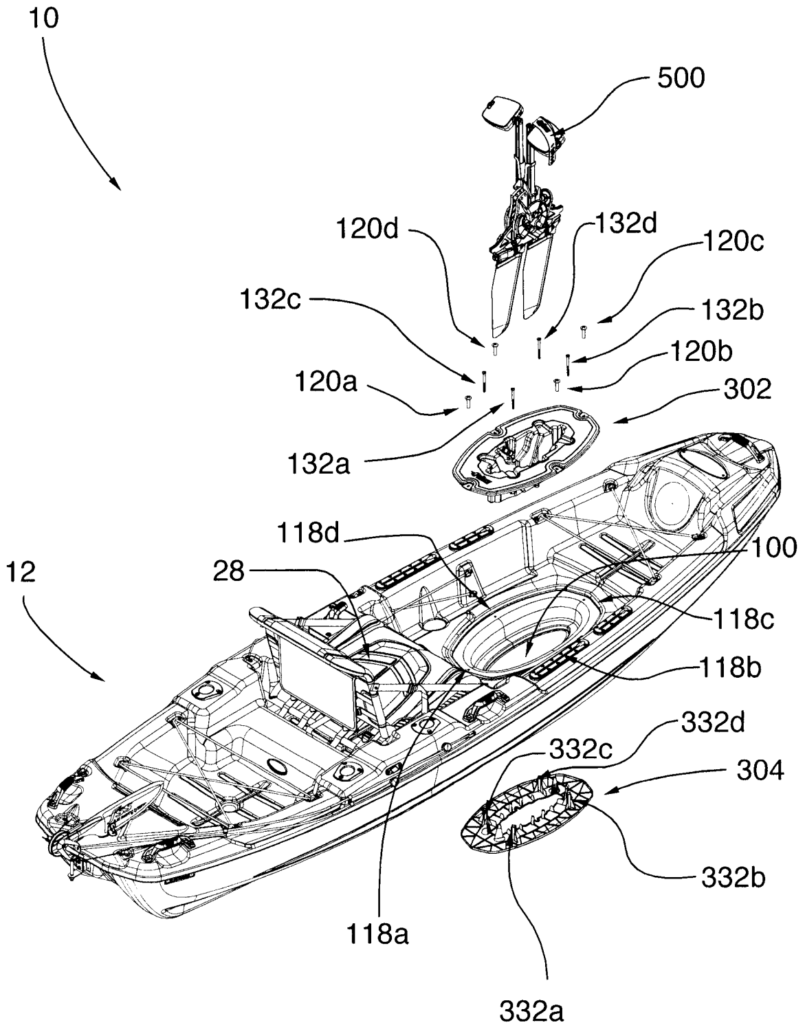
FIG.31
