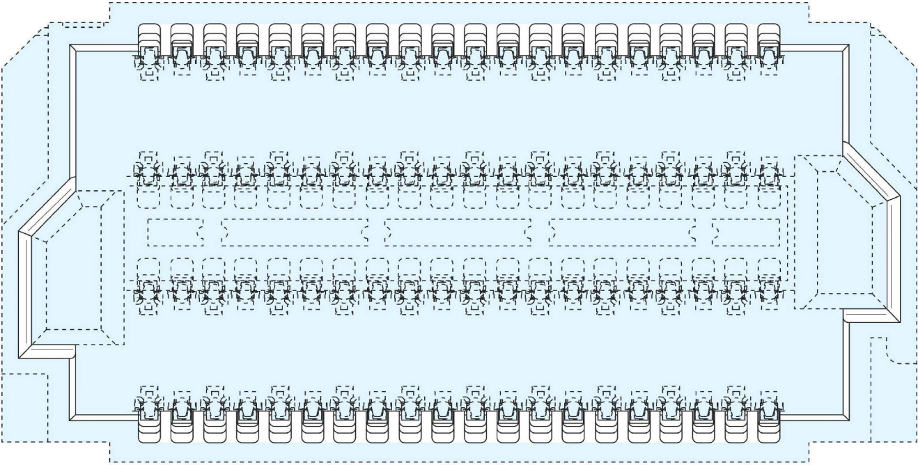
【俯視圖】
