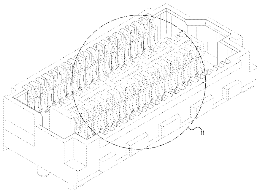
【立體圖1】
