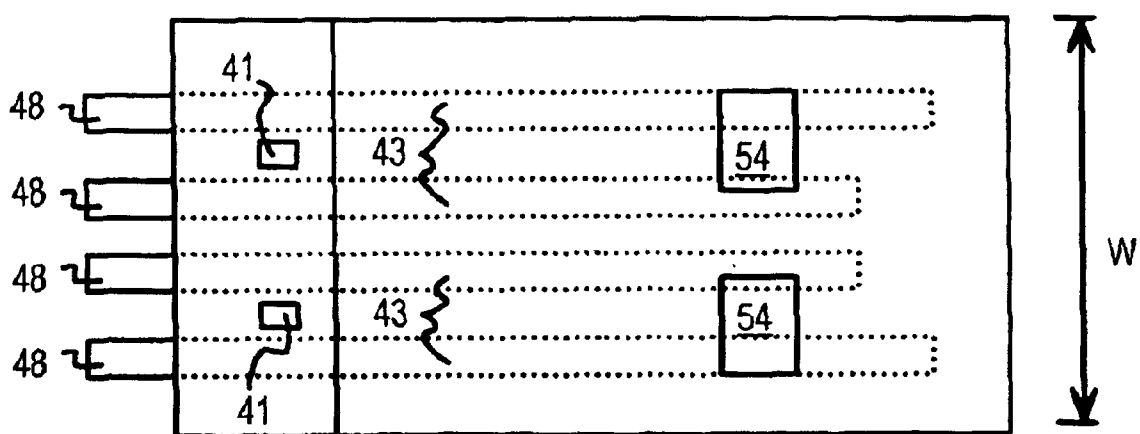
BOTTOM VIEW FIG. 5E
