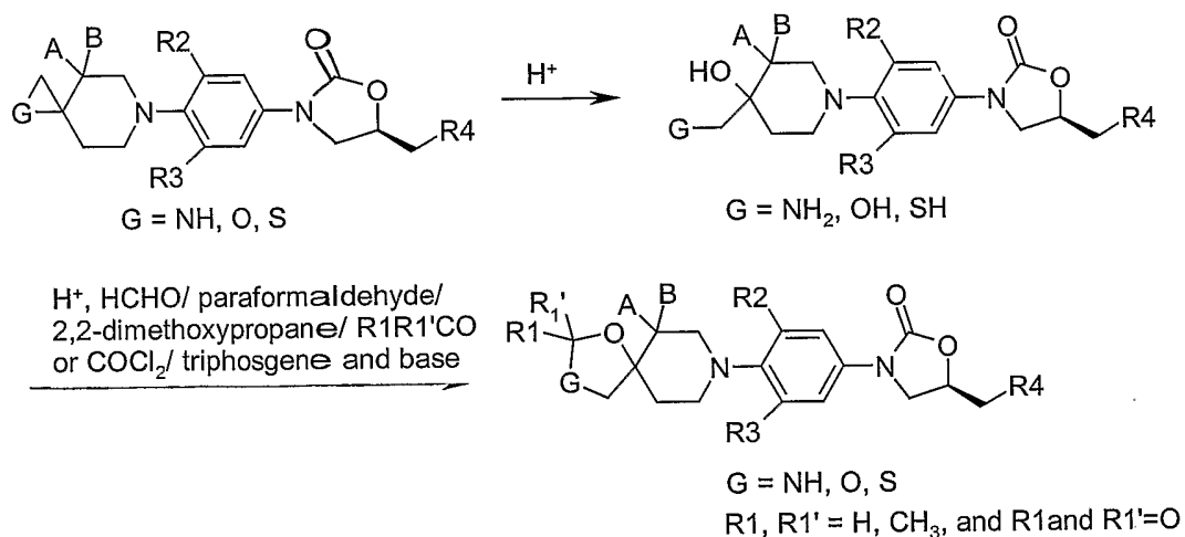
Scheme-4
