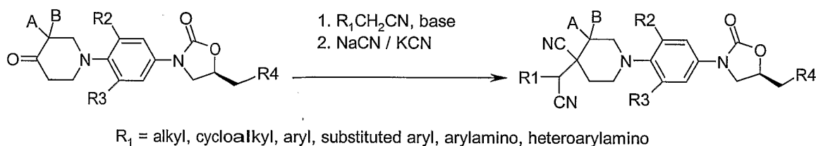
Scheme-17
