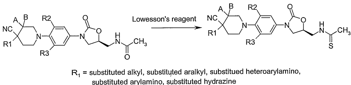
Scheme-19
