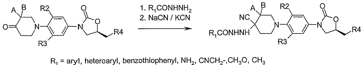
Scheme-18
