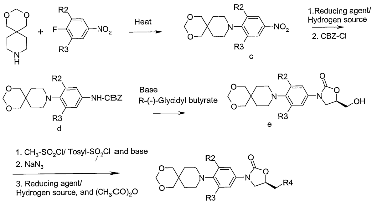
Scheme-6
