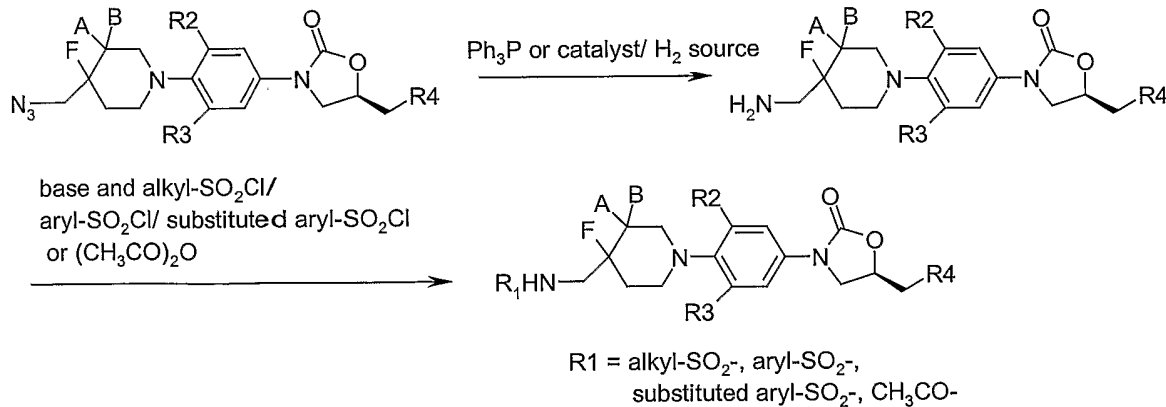
Scheme-14
