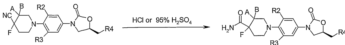
Scheme-13
