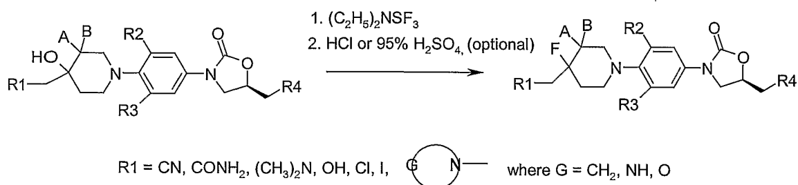
Scheme-11
