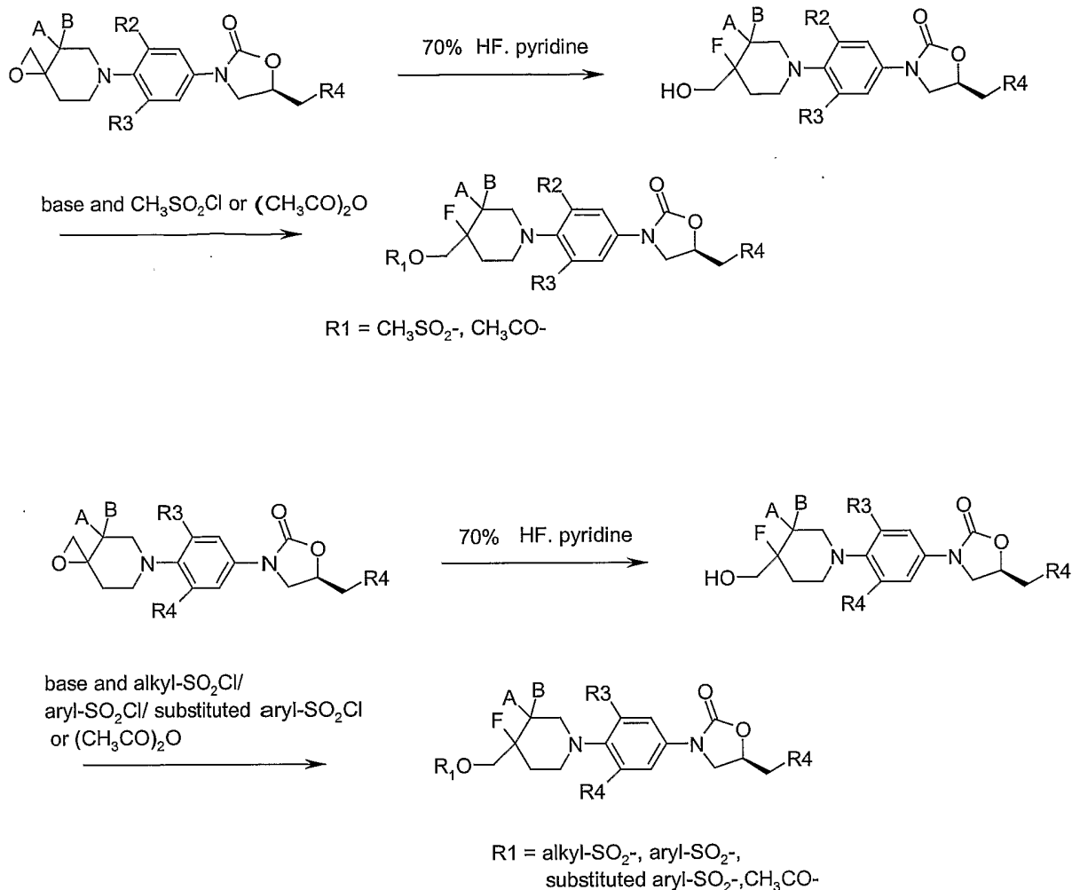
Scheme-12
