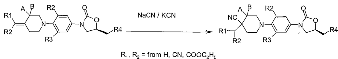
Scheme-16
