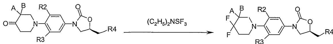
Scheme-10
