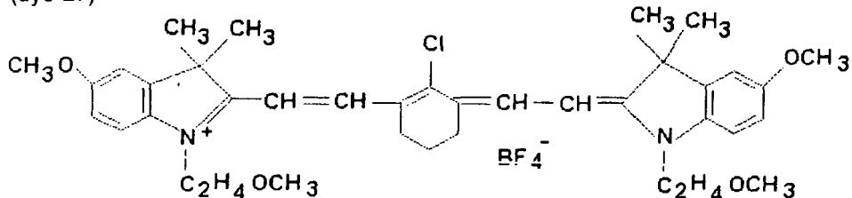
(dye 28)
