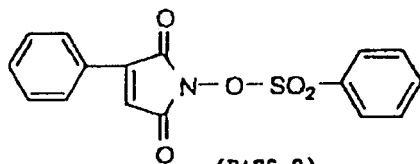
(PAG6-9)
