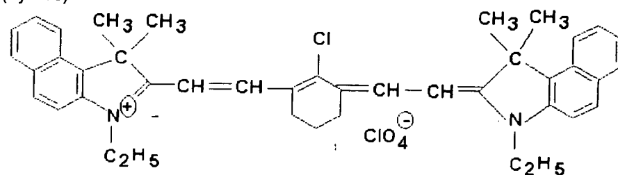
(dye 15)
