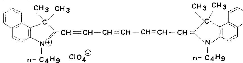
(dye 10)
