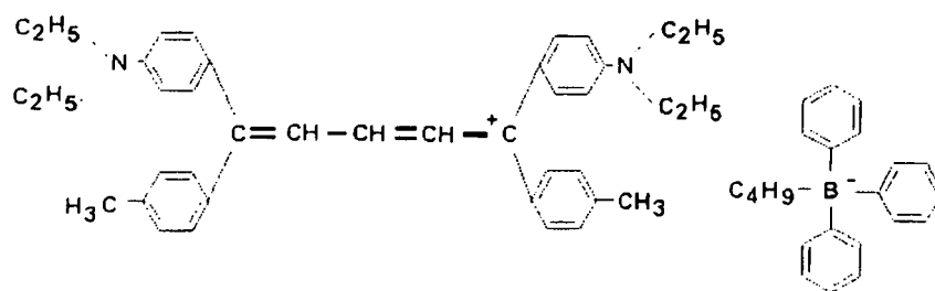
(dye 6)
