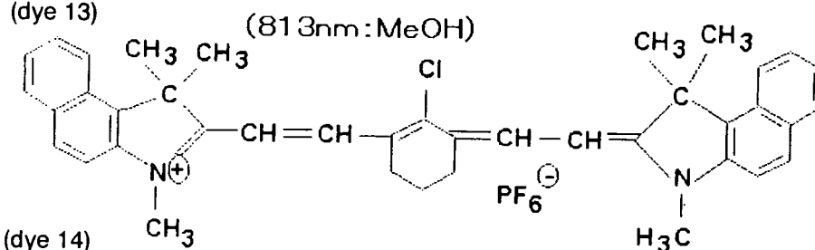
(dye 13)
