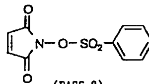
(PAG6-8)
