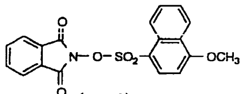
(PAG6-6)
