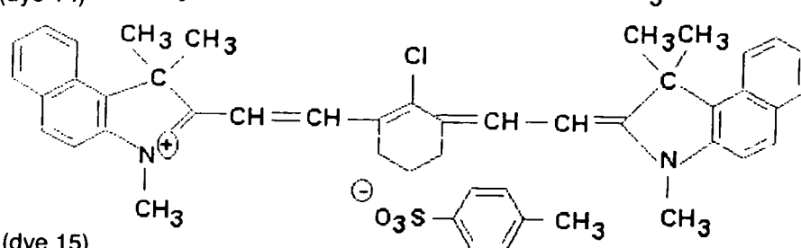
(dye 14)
