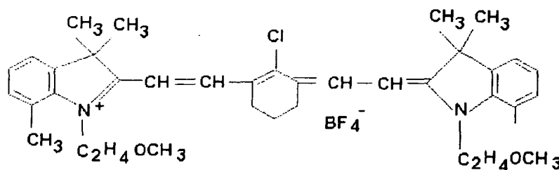
(dye 30)
