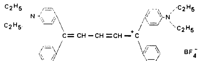
(dye 1)
