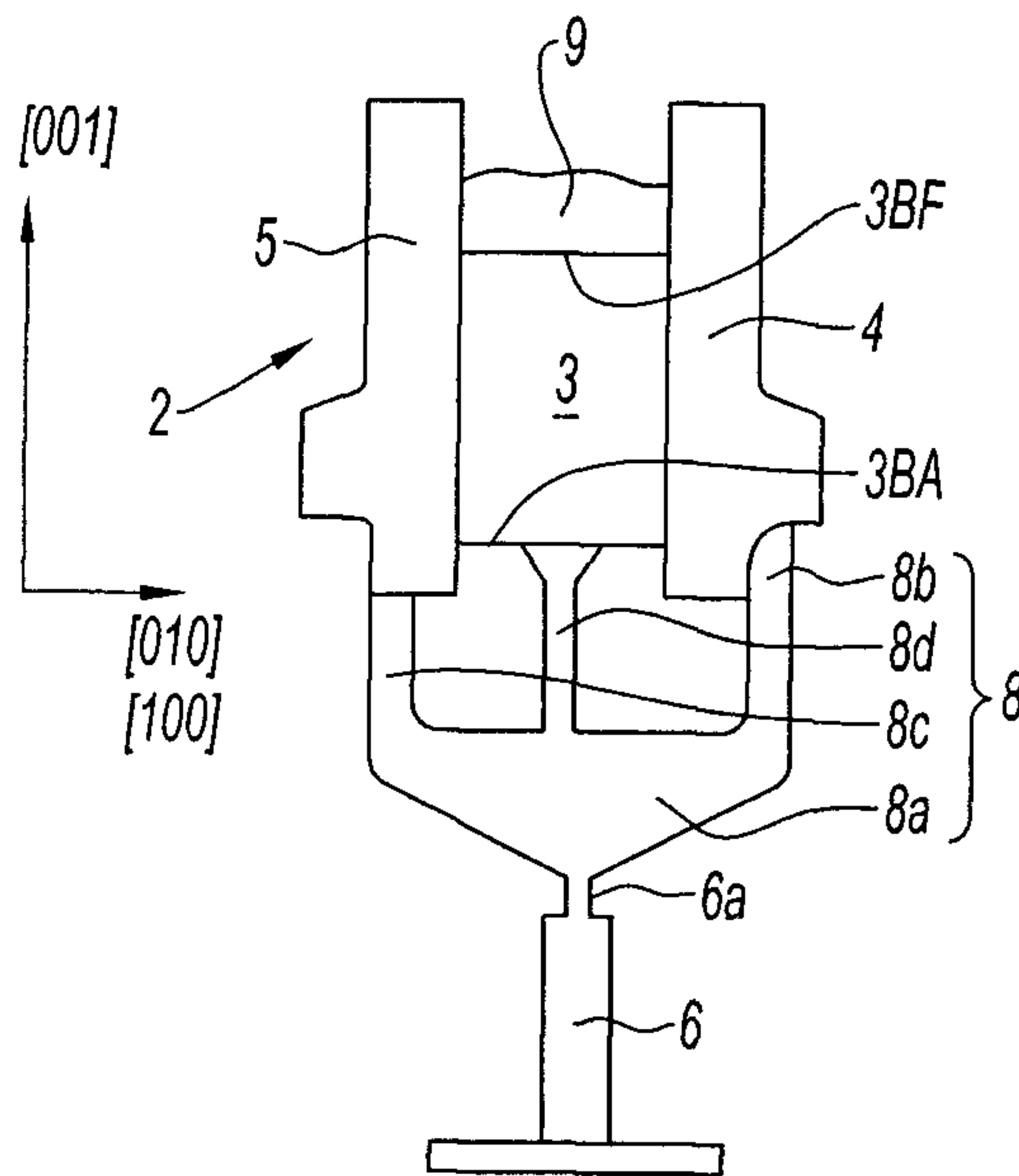
Fig. 1 ART ANTERIEUR
