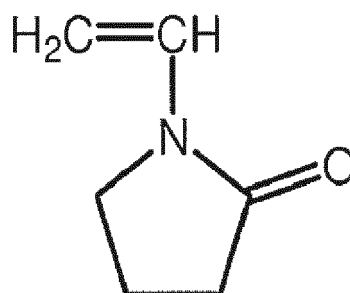
Vinylpyrrolidone
