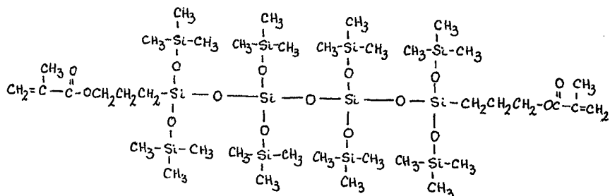
1,7-Bis( \gamma -methacryloxypropyl)-1,1,3,3,5,5,7,7-octa(trimethylsiloxy)tetra siloxane
