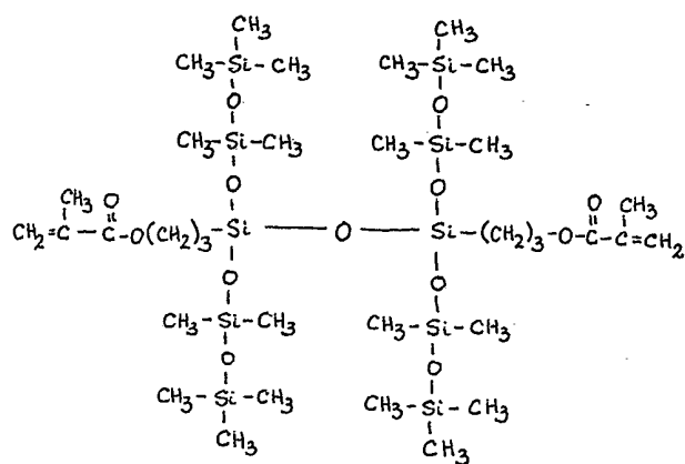
1,3-Bis( \gamma -methacryloxypropyl)-1,1,3,3-tetra(pentamethyl disiloxanyl)disiloxane
