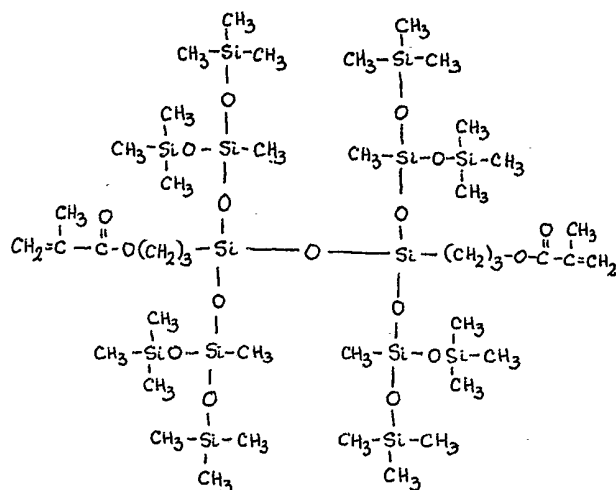
1,3-Bis( \gamma -methacryloxypropyl)-1,1,3,3-tetra[Bis(trimethylsiloxy)methyl siloxanyl]disiloxane
