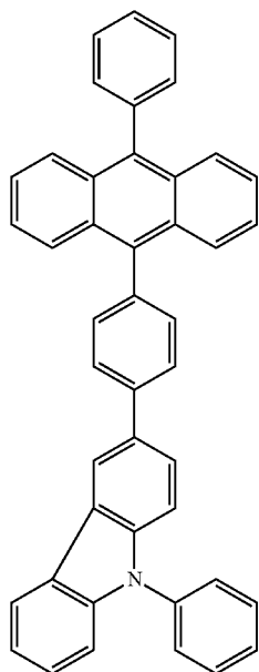
PCzPA
