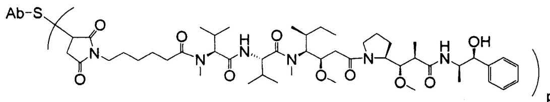
Ab-MC-MMAE
