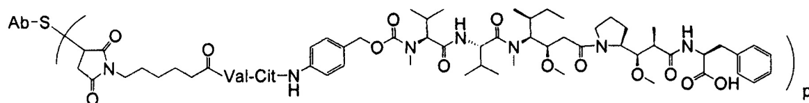
Ab-MC-vc-PAB-MMAF
