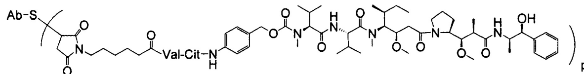
Ab-MC-vc-PAB-MMAE
