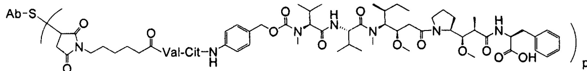
Ab-MC-vc-PAB-MMAF
