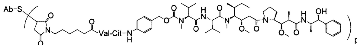
Ab-MC-vc-PAB-MMAE
