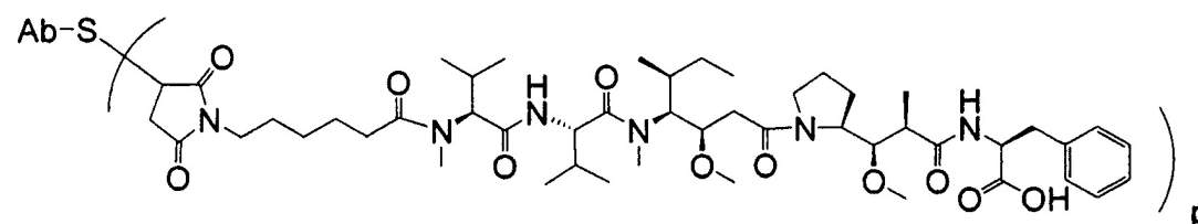
Ab-MC-MMAF
