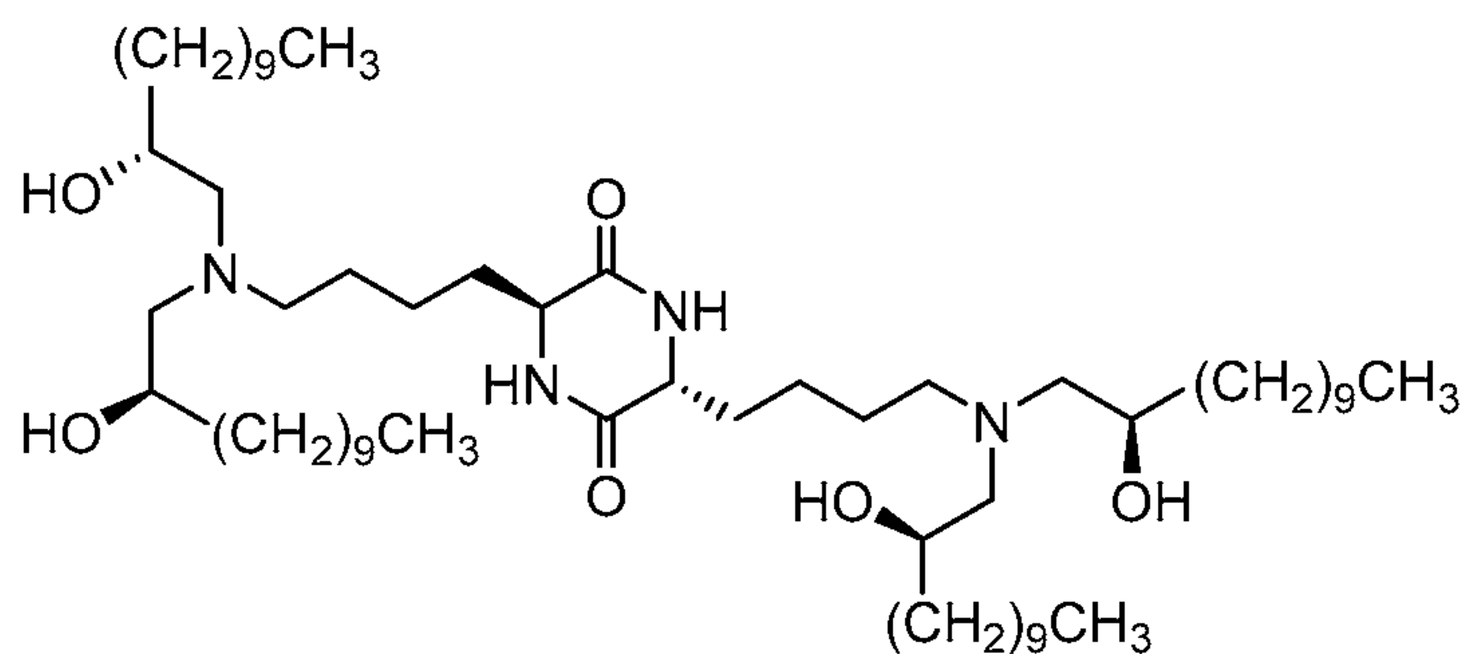
I.a.i ( i.e. , R4-SR-cKK-E12 )
