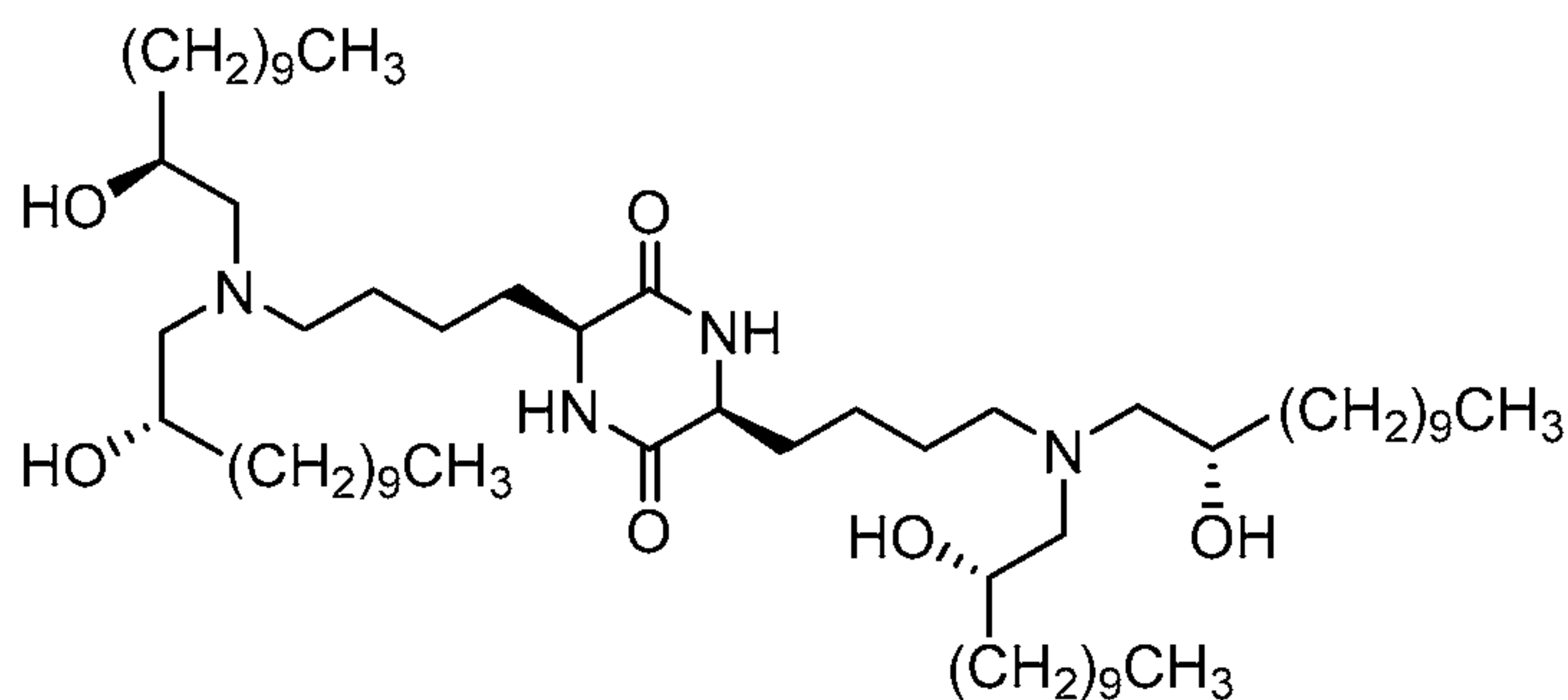
I.b.1.ii ( i.e. , S4-SS-cKK-E12 )
