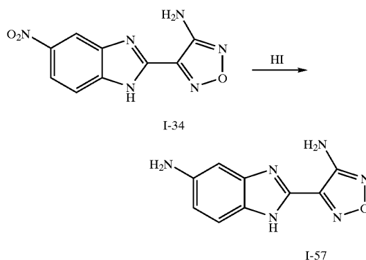
Scheme XXVII:
