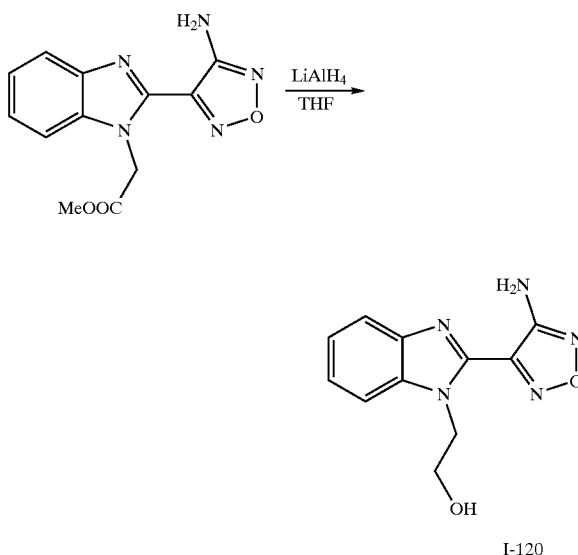
Scheme VIII:
