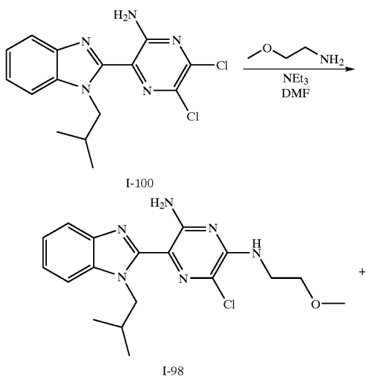
Scheme XIV:
