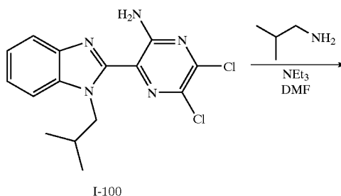
Scheme XIII:
