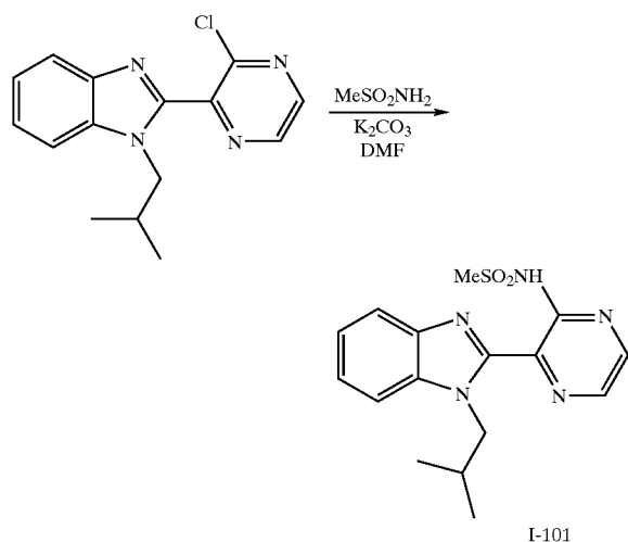
Scheme XXIII:
