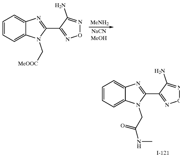
Scheme VII:
