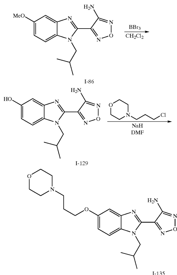
Scheme XXVI:
