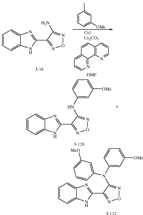
Scheme XI:
