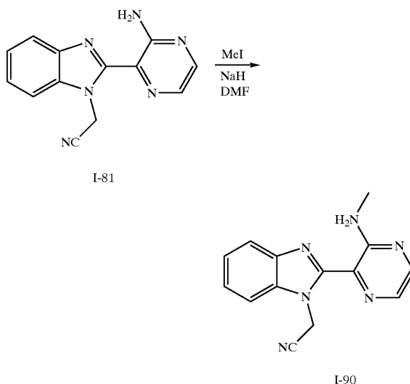
Scheme XXIV:
