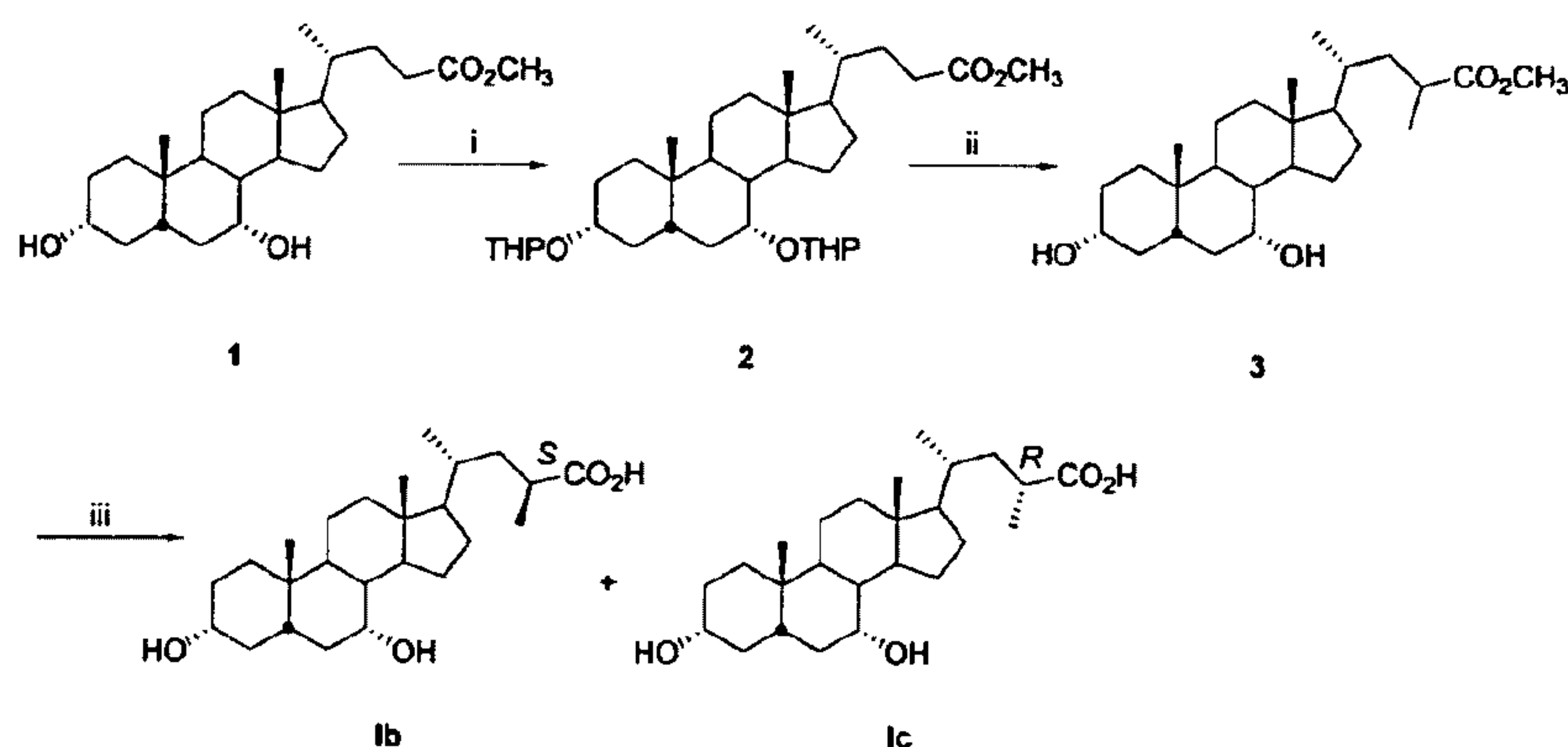
Scheme 1. (i) 3,4-DHP, p -TSA, dioxane, r.t.; (ii) a) LDA, CH 3 I, -78 °C; b) HCl, CH 3 OH, r.t.; (iii) NaOH, CH 3 OH, reflux.
