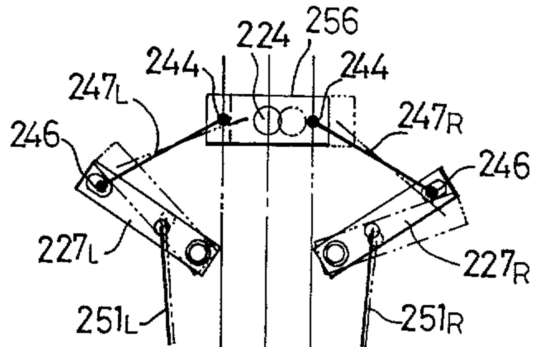
FIG. 19A V=5.2km/h
