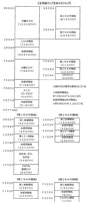
【主制御チップメモリマップ構成図】
