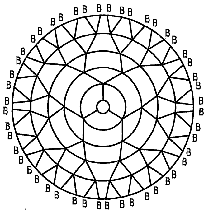
DENDRIMER
