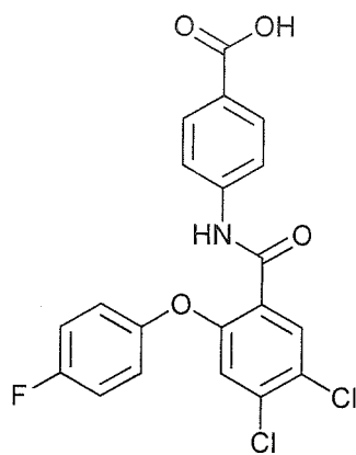
4-(4,5-dichloro-2-(4-fluorophenoxy)benzamido)benzoic acid;
