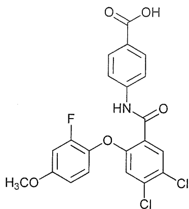
4-(4,5-dichloro-2-(2-fluoro-4-methoxyphenoxy)benzamido)benzoic acid;
