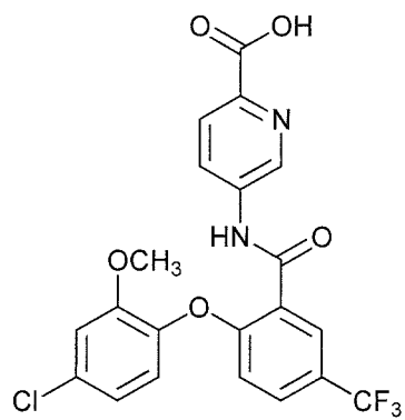
5-(2-(4-chloro-2-methoxyphenoxy)-5-(trifluoromethyl)benzamido)picolinic acid;
