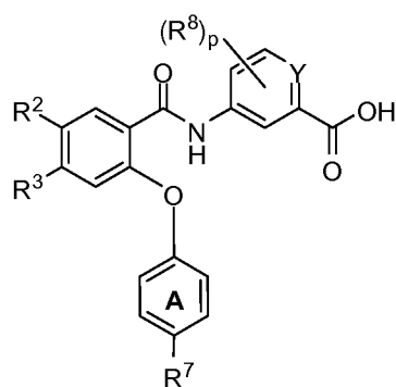
I'-L
