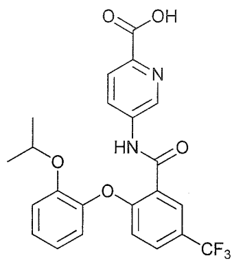
5-(2-(2-isopropoxyphenoxy)-5-(trifluoromethyl)benzamido)picolinic acid;
