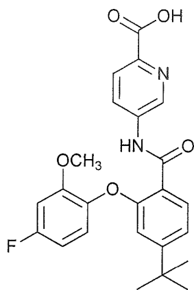
5-(4-(tert-butyl)-2-(4-fluoro-2-methoxyphenoxy)benzamido)picolinic acid;
