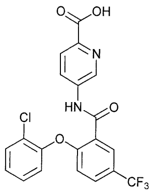
5-(2-(2-chlorophenoxy)-5-(trifluoromethyl)benzamido)picolinic acid;
