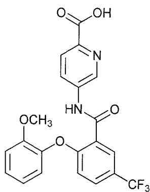
5-(2-(2-methoxyphenoxy)-5-(trifluoromethyl)benzamido)picolinic acid;
