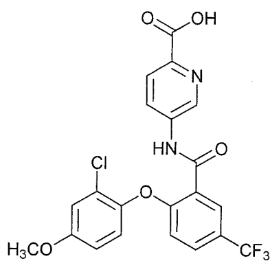
5-(2-(2-chloro-4-methoxyphenoxy)-5-(trifluoromethyl)benzamido)picolinic acid;
