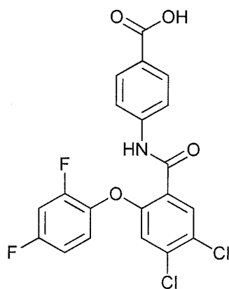
4-(4,5-dichloro-2-(2,4-difluorophenoxy)benzamido)benzoic acid;
