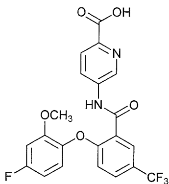
5-(2-(4-fluoro-2-methoxyphenoxy)-5-(trifluoromethyl)benzamido)picolinic acid;
