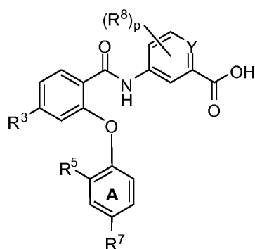
I'-F
