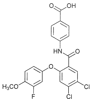
4-(4,5-dichloro-2-(3-fluoro-4-methoxyphenoxy)benzamido)benzoic acid;
