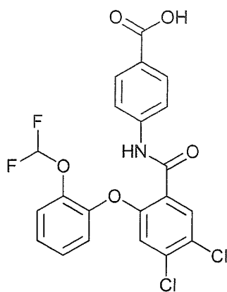
4-(4,5-dichloro-2-(2-(difluoromethoxy)phenoxy)benzamido)benzoic acid;
