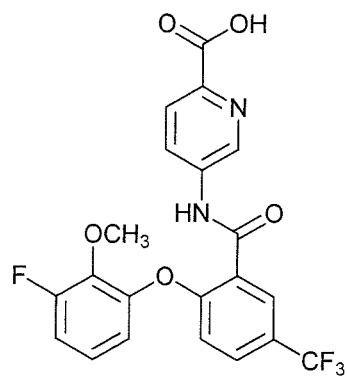
5-(2-(3-fluoro-2-methoxyphenoxy)-5-(trifluoromethyl)benzamido)picolinic acid;
