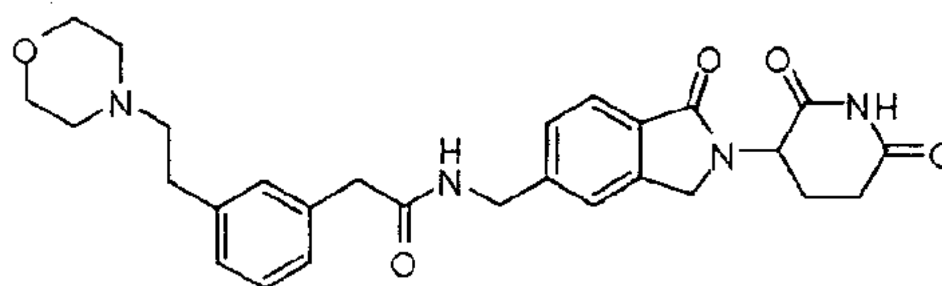
N-((2-(2,6-dioxopiperidin-3-yl)-1-oxoisindolin-5-yl)methyl)-2-(3-(2-morpholinoethyl)phenyl)acetamide;
