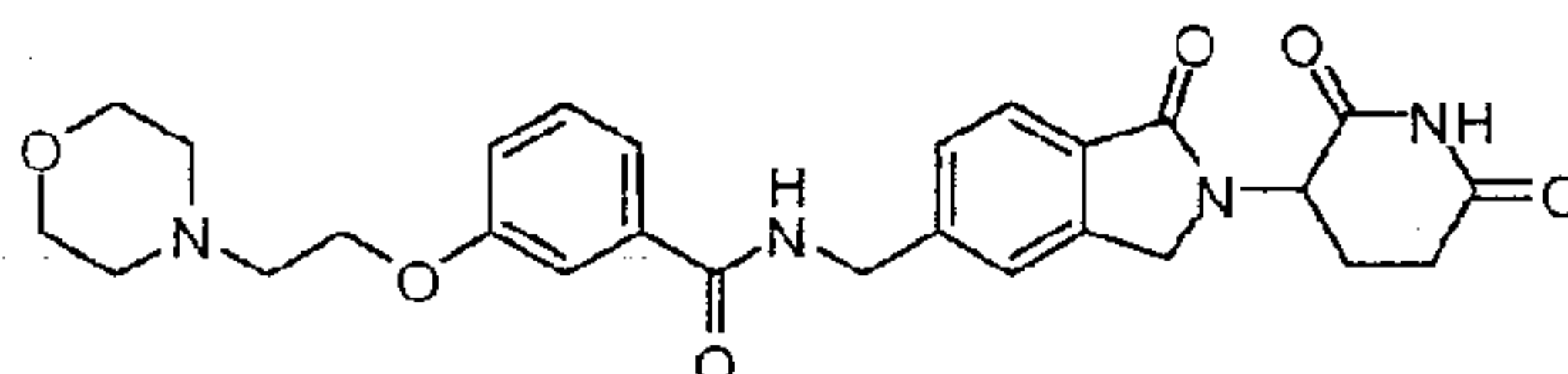
N-((2-(2,6-dioxopiperidin-3-yl)-1-oxoisindolin-5-yl)methyl)-3-(2-morpholinoethoxy)benzamide;
