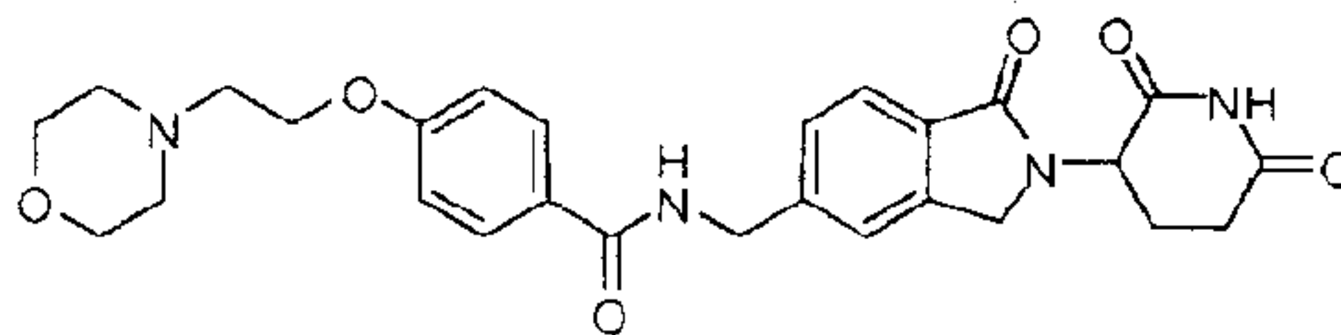
N-((2-(2,6-dioxopiperidin-3-yl)-1-oxoisindolin-5-yl)methyl)-4-(2-morpholinoethoxy)benzamide;
