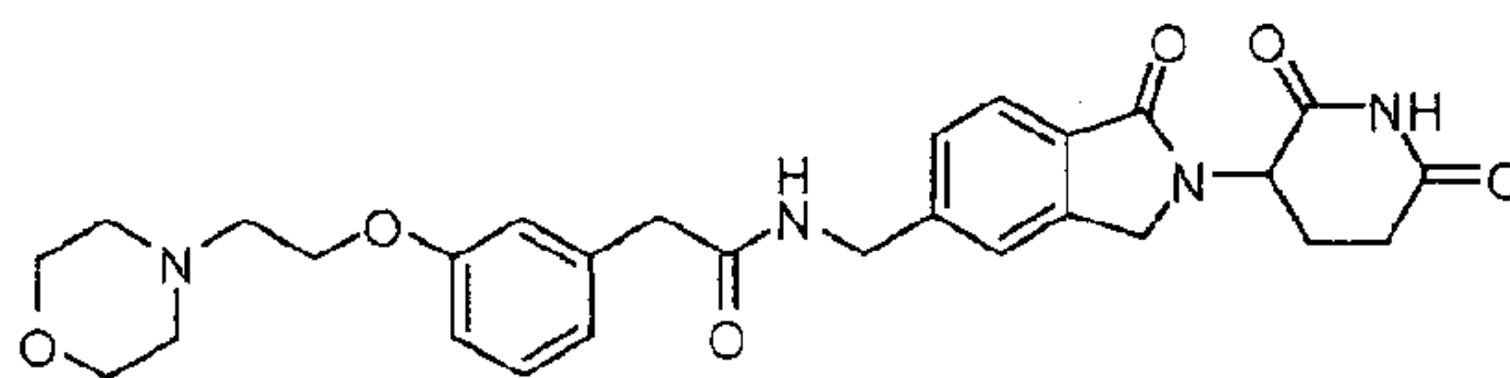
N-((2-(2,6-dioxopiperidin-3-yl)-1-oxoisindolin-5-yl)methyl)-2-(3-(2-morpholinoethoxy)phenyl)acetamide;
