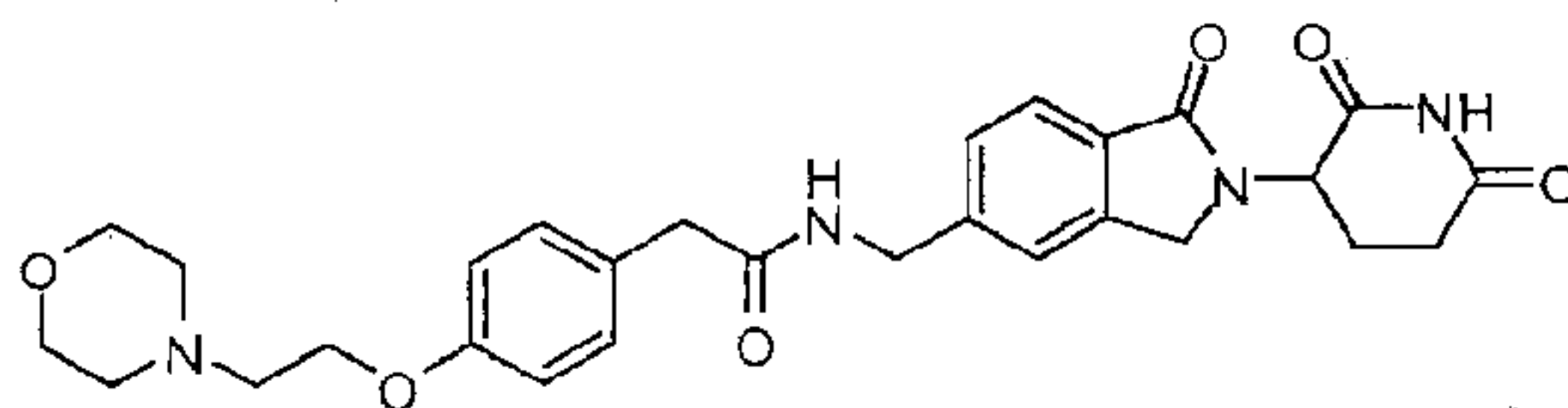
N-((2-(2,6-dioxopiperidin-3-yl)-1-oxoisindolin-5-yl)methyl)-2-(4-(2-morpholinoethoxy)phenyl)acetamide;
