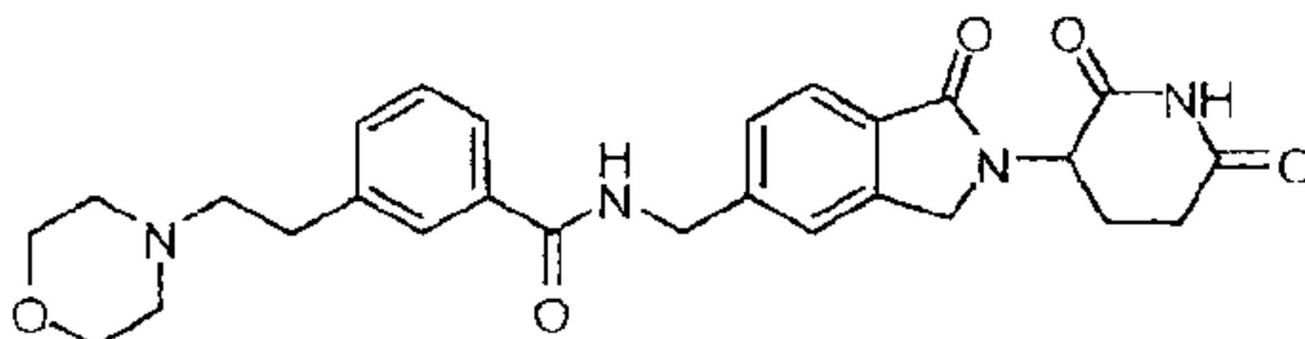
N-((2-(2,6-dioxopiperidin-3-yl)-1-oxoisindolin-5-yl)methyl)-3-(2-morpholinoethyl)benzamide;
