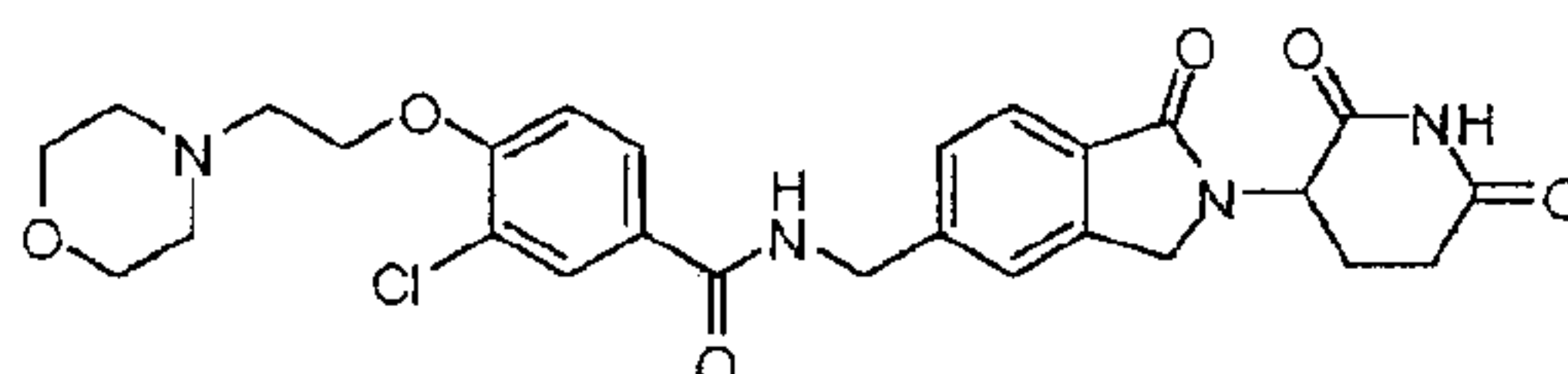
3-chloro-N-((2-(2,6-dioxopiperidin-3-yl)-1-oxoisindolin-5-yl)methyl)-4-(2-morpholinoethoxy)benzamide;
