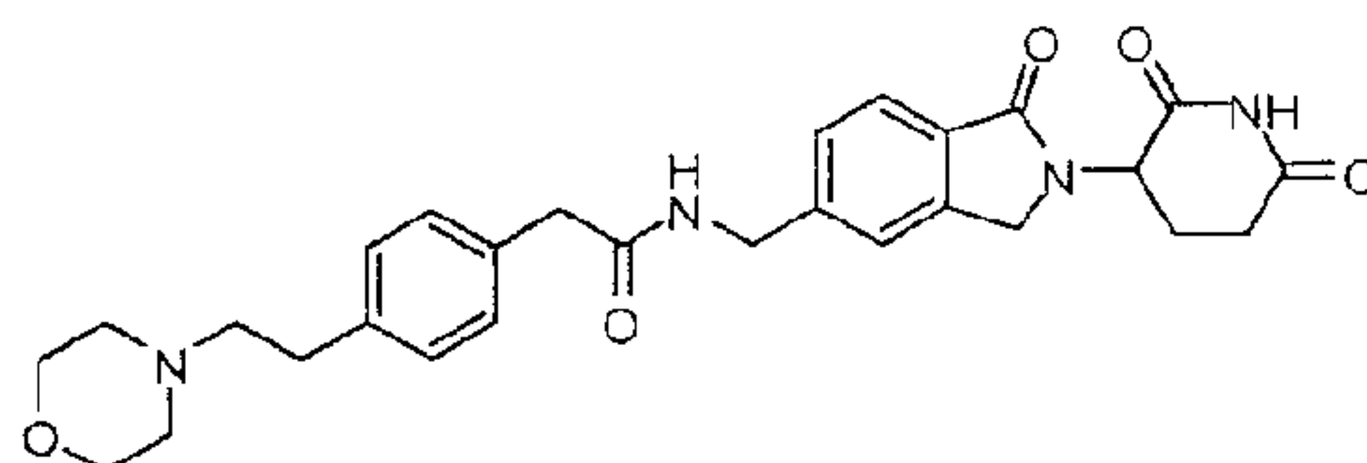
N-((2-(2,6-dioxopiperidin-3-yl)-1-oxoisindolin-5-yl)methyl)-2-(4-(2-morpholinoethyl)phenyl)acetamide;
