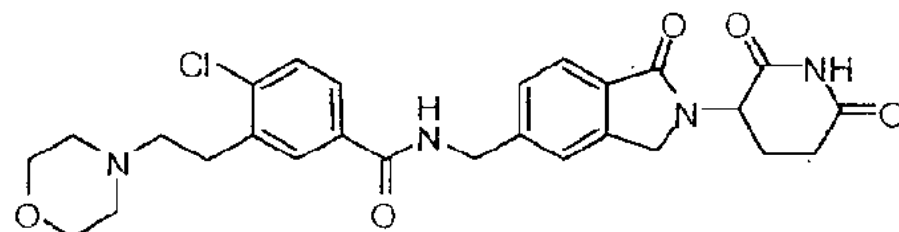
4-chloro-N-((2-(2,6-dioxopiperidin-3-yl)-1-oxoisindolin-5-yl)methyl)-3-(2-morpholinoethyl)benzamide;
