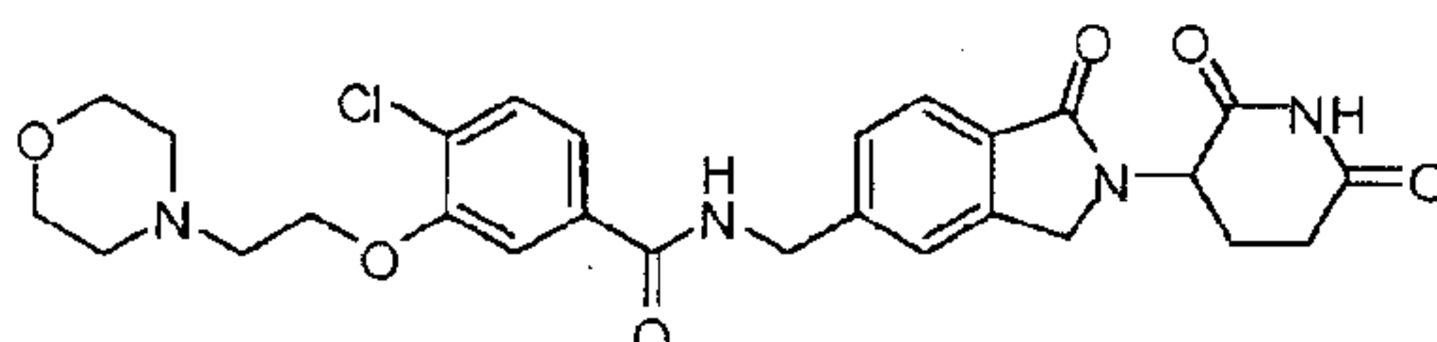
4-chloro-N-((2-(2,6-dioxopiperidin-3-yl)-1-oxoisindolin-5-yl)methyl)-3-(2-morpholinoethoxy)benzamide.
