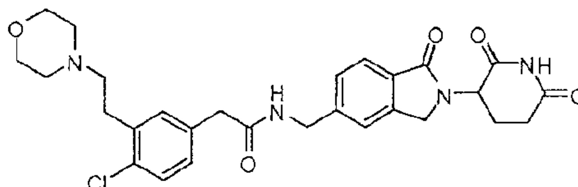
2-(4-chloro-3-(2-morpholinoethyl)phenyl)-N-((2-(2,6-dioxopiperidin-3-yl)-1-oxoisindolin-5-yl)methyl)acetamide;
