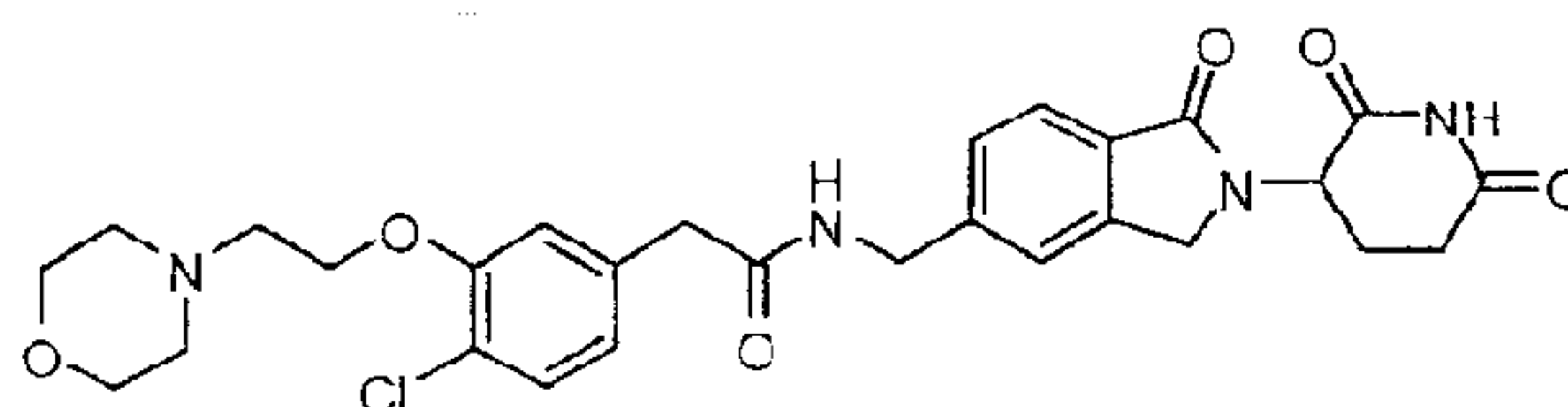
2-(4-chloro-3-(2-morpholinoethoxy)phenyl)-N-((2-(2,6-dioxopiperidin-3-yl)-1-oxoisindolin-5-yl)methyl)acetamide;
