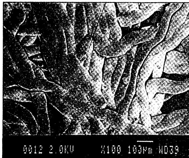
FIG. 3 STANDARD POLYAMIDE 6,6
