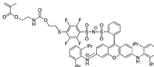
色素単量体M-27（染料ai）
