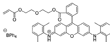
色素単量体M-29（染料ak）
