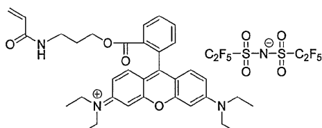
色素単量体M-25（染料ag）
