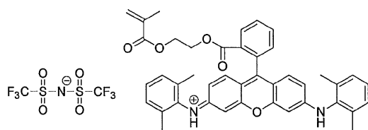
色素単量体M-24（染料af）
