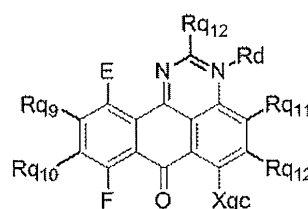
一般式 (A Q - 3)
