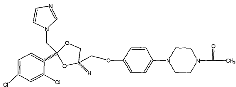
KETOCONAZOLE
