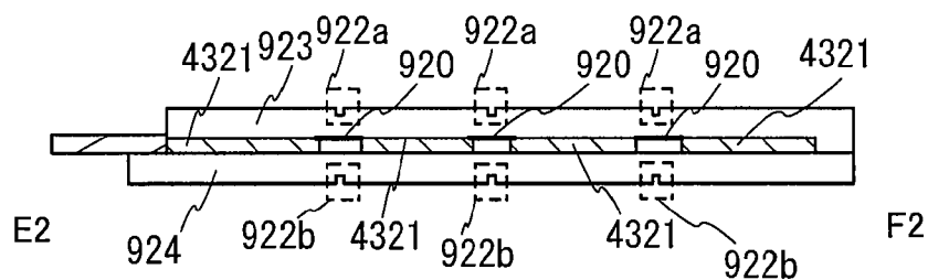
FIG. 10C
