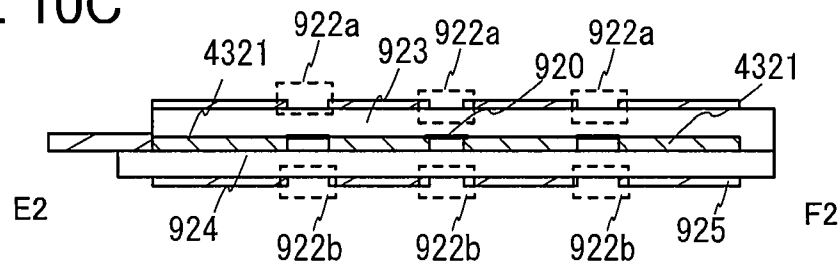
FIG. 10C
